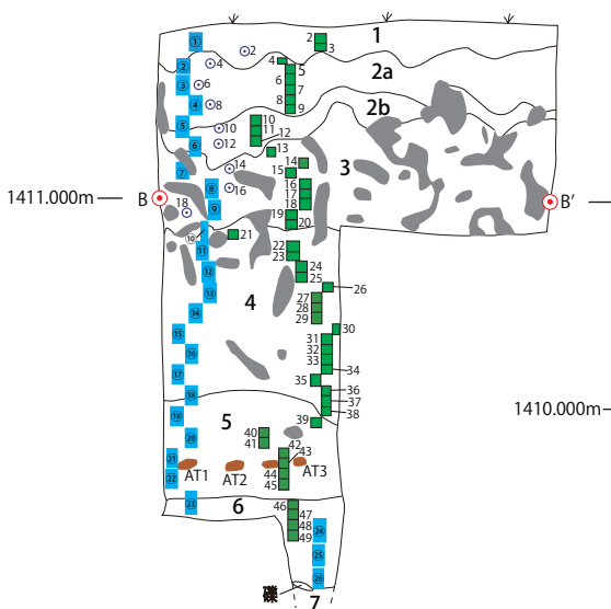
TP-2 南壁セクション
