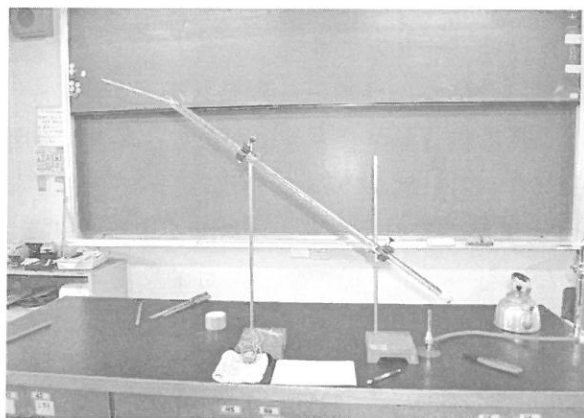
図1 蛍光管の下部を加熱する実験装置
