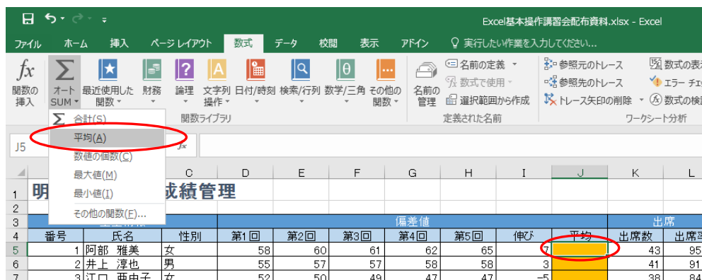
図 4-1 平均
