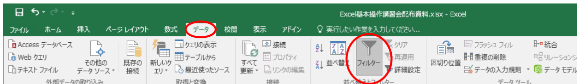
図 6-4 フィルター
